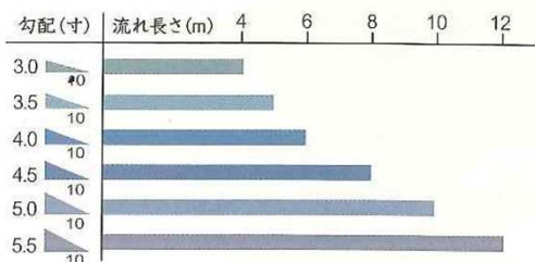
標準屋根勾配と流れ長さ
