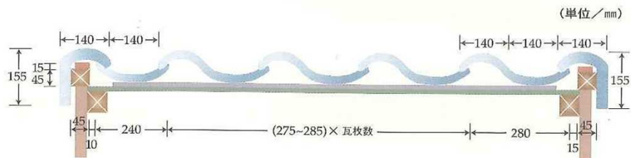
エル形袖／横の割付寸法
